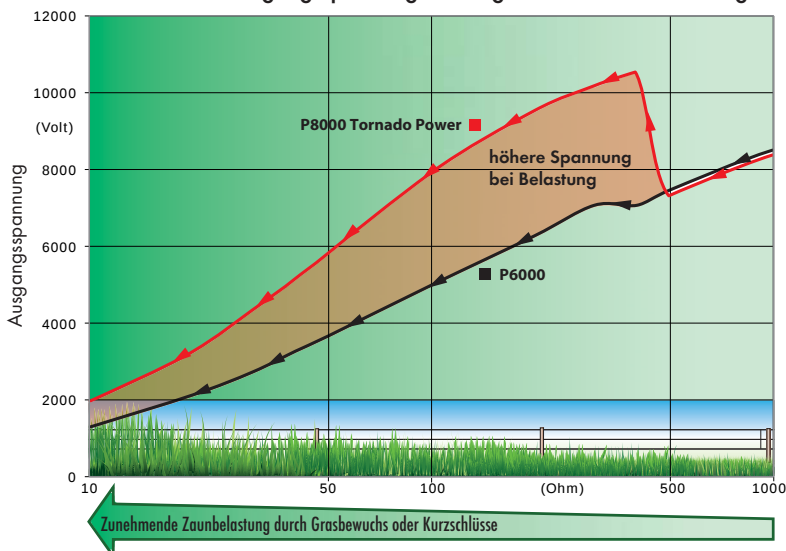
Vergleich P8000 Tornado Power mit P6000: Verlauf der Ausgangsspannung bei steigender Bewuchsbelastung
