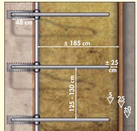
Maße Liegeboxenmontage Classic als Tiefbox für Großvieh (Alle Maße sind unverbindliche Richtmaße!)
