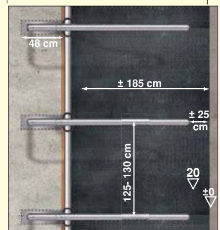
Maße Liegeboxenmontage Classic als Hochbox für Großvieh (Alle Maße sind unverbindliche Richtmaße!)
