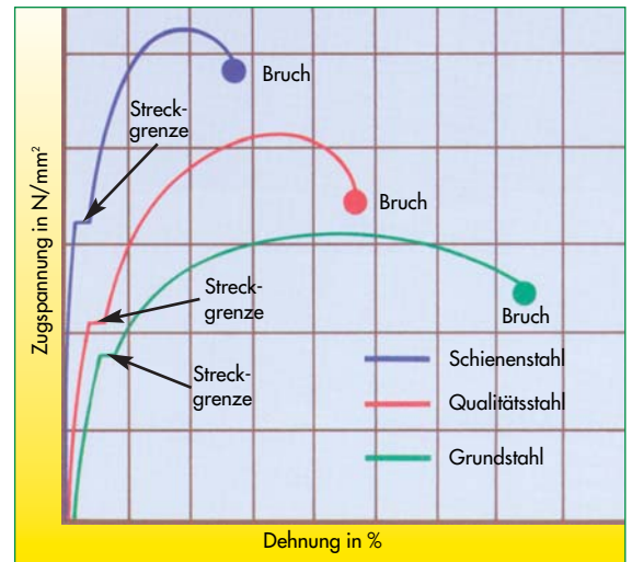
Spannungs-Dehnungsdiagramm verschiedener Stähle Schienenstahl einer der am höchsten zu beanspruchenden Stahlarten. Schienenstahl verfügt über höchste Steifheit und verkräftet schwerste Beanspruchung mit minimalster Verformung.
