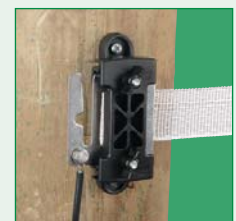
Breitband-Zugisolator: Querverbindung von Bändern
